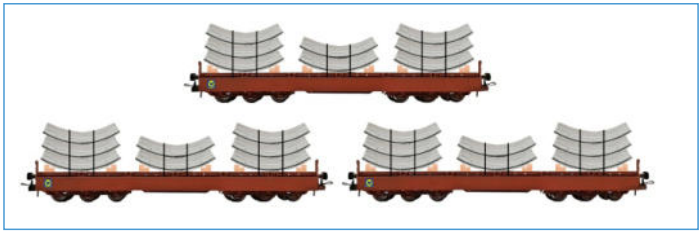
6-achsiges Schwerlastwagen-Set Bauart Samms-u 454 der DB AG (Epoche VI) 30 Jahre ICE 1991 - 2021 Tunnelbauzug der Walter Bau AG
