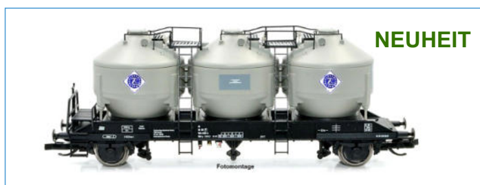
2-achsiges Silowagen Bauart Udd-y der DR VEB Zuckerfabrik Nauen (Epoche IV) zum Transport von Zucker NW 52110 DC 2L TT 54,90 €
