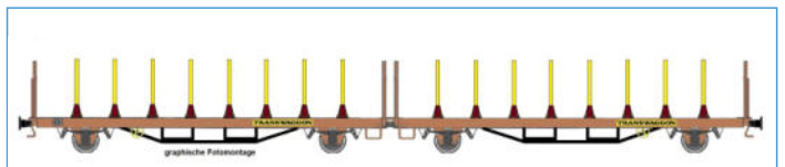
4achsige Flachwagen-Doppelereinheit Bauart Laas 1 der Fa. Transwaggon eingestellt bei der DB AG (Ep.V/VI) rotbraun einfarbig, unbel., ExTe-Rungen, gelb
