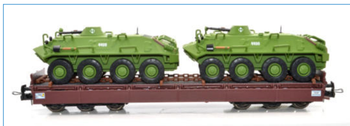
6-achsiger Schwerlastwagen Bauart Sas 4850 der DR (Epoche IV) Militärverkehr, Ursprungsausführung beladen mit Schützenpanzern BTR 60 PB, polnisches Militär
